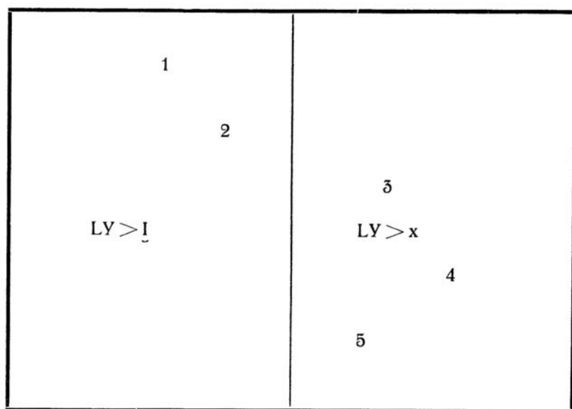
3.—Soluciones de Ly
