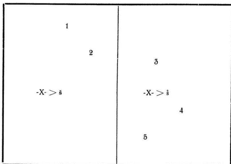
8.—Soluciones de -x-
