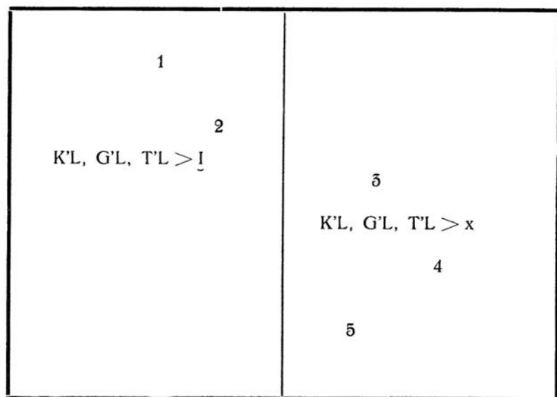
4.—Soluciones de K'L, G'L, T'L
