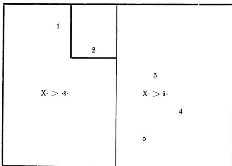
7.—Soluciones de x-
